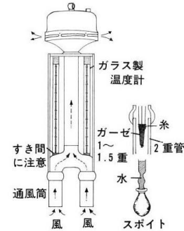
図 1. アスマン乾湿計
