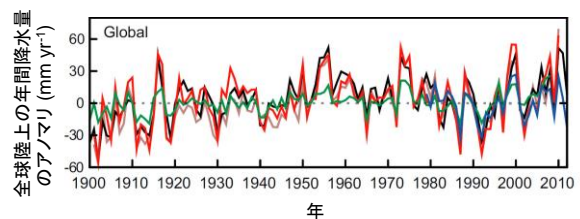
図 5. 全球陸上の年間降水量のアノマリ 1981-2000 年に対する相対値 (IPCC, 2013)
