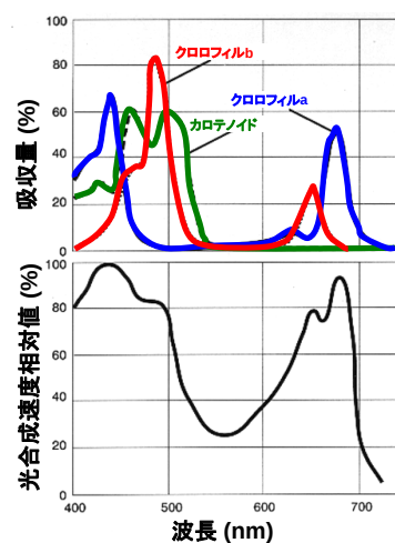
図3 植物の吸光特性の典型値 (Wikipedia より)
