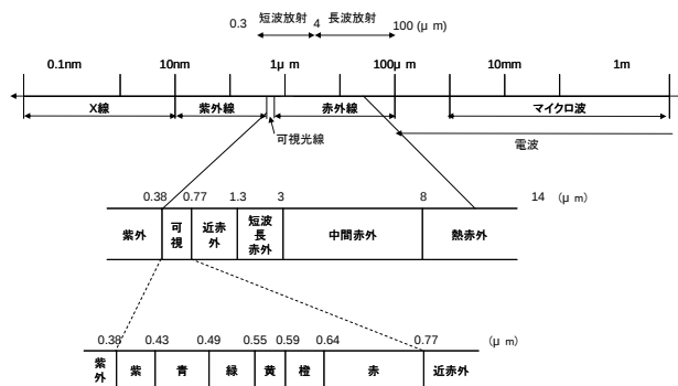
図1 電磁波の名称と波長 (図解リモートセンシングより作成)
