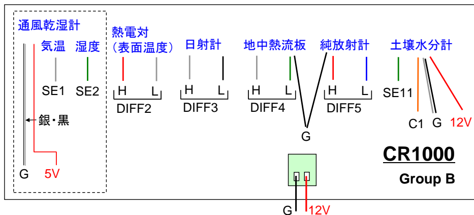
図 3. グループ B のロガー配線図
