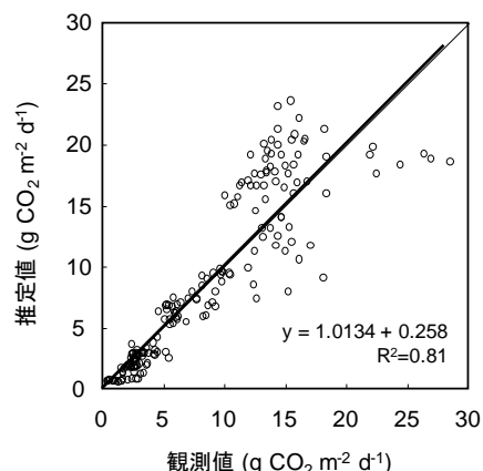
図 8. 指数回帰式による推定値と観測値による土壤呼吸速度の比較。細線は 1:1 線、太線は両者の直線回帰式を表す。
