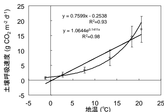
図7. 地温に対する土壌呼吸速度の関係。データは5℃毎の地温のクラスにまとめられている。
