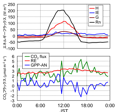
図 2 フラックスの平均日変化パターン (期間：2014.10.30–2014.11.28)
