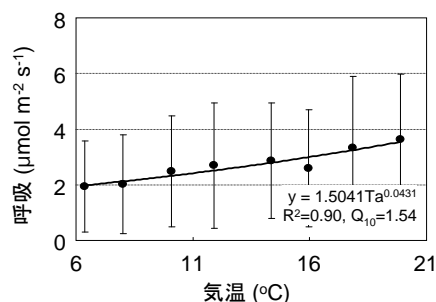
図 1 夜間の CO 2 フラックスと気温の関係 (期間 : 2014.10.30 – 2014.11.28)
