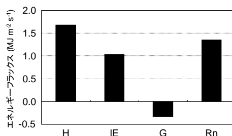
図 4 エネルギーフラックスの積算値 (2014.10.30–2014.11.28)
