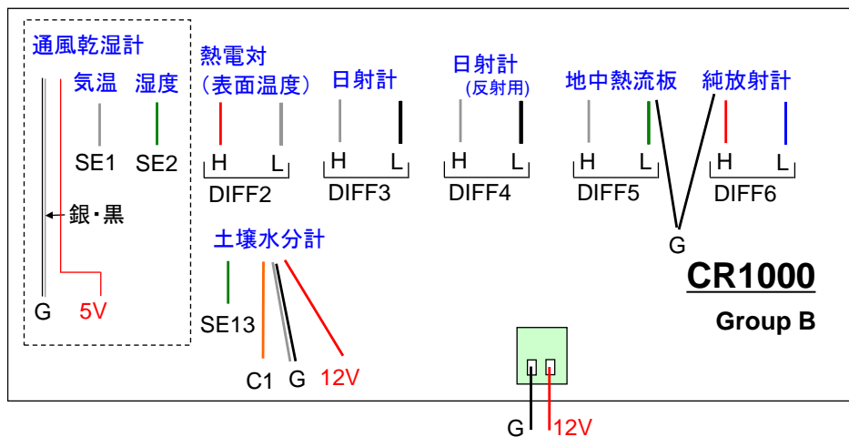
図 3. グループ B のロガー配線図
