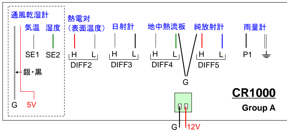
図 2. グループ A のロガー配線図
