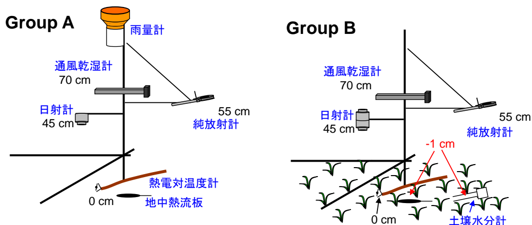
図 1. 測定機器の取り付けについての模式図
