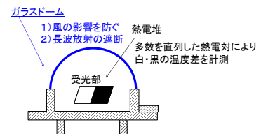
図 8. 熱電式日射計の模式図
