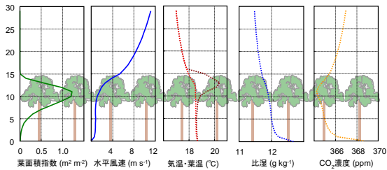
図2 風速が2倍になったときは？ 点線は1倍の風速時の鉛直プロファイル
