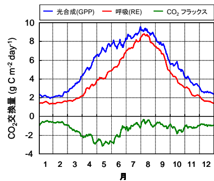
図 9 ヒノキ林の CO_2 交換量 2000~2007 年の平均的な季節変化
