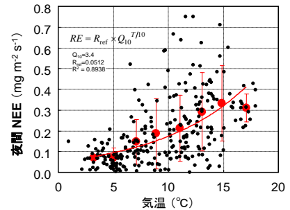
図 7 夜間の CO_2 フラックスと気温の関係
