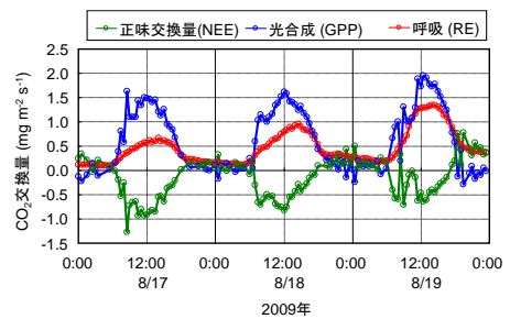
図 8 ヒノキ林における CO_2 フラックス、光合成、呼吸の日変化
