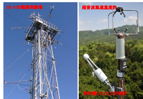
写真 1 ヒノキ林の観測用鉄塔と渦相関法測定システム
