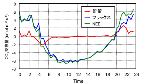
図5 フラックスと貯留の関係 アラスカのクロトウヒ林の場合
